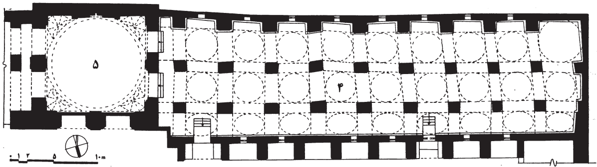
نقشه ۱. پلان مسجد جامع ارومیه (مأخذ: حاجی قاسمی، ۱۳۸۳).
